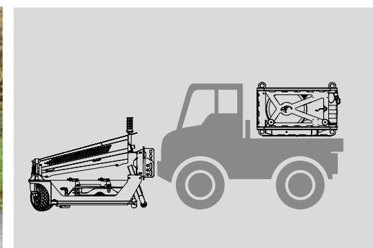
Opbouwframe met gastank op werktuigendrager
